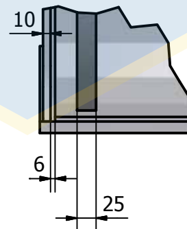
C ( 0,18 : 1 )
